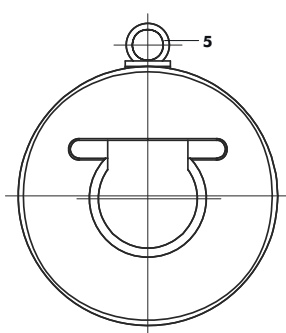
Исполнение из 2 частей DN 40-300 мм, 1/2"-12"
