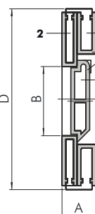
Исполнение из 3 частей DN 350-600 мм, 14"-24"
