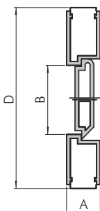
Исполнение из 2 частей DN 40-300 мм, 1/2"-12"
